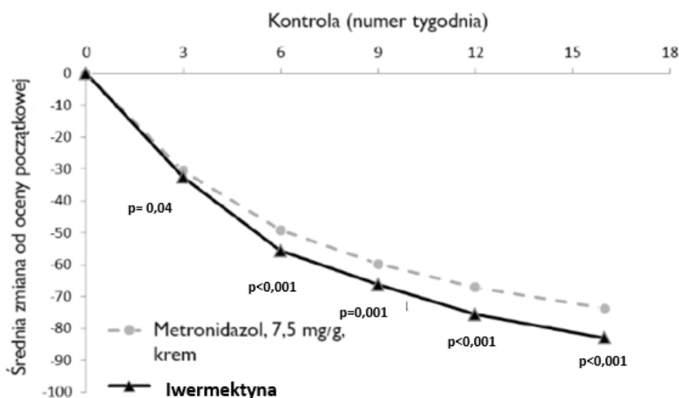
Rycina 5: Średnia zmiana procentowa w czasie w kolejnych tygodniach
